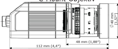
C-Mount-Objektiv
